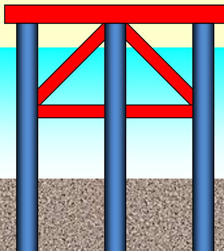
【中間ブレス工法】
