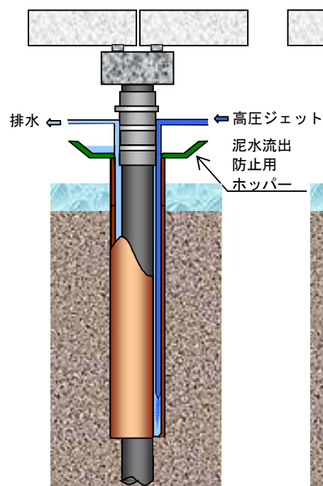
⑥高圧ジェットによる洗浄
