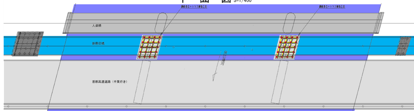
平面図 S=1/400
