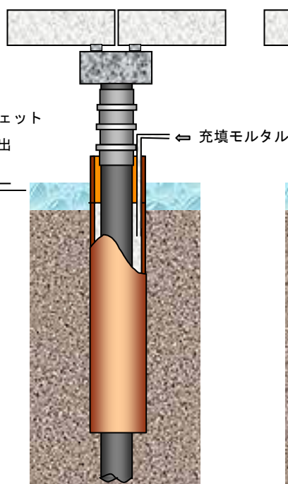
⑦充填モルタルの充填
