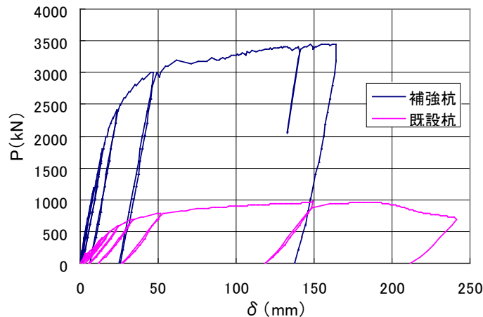
荷重-変位関係
