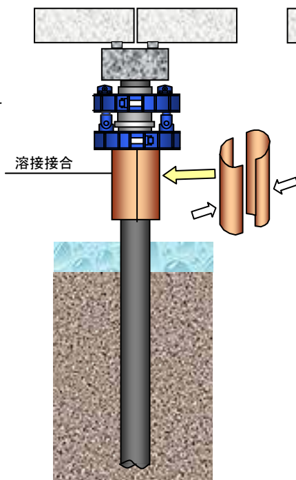
②圧入装置と補強鋼板の設置
