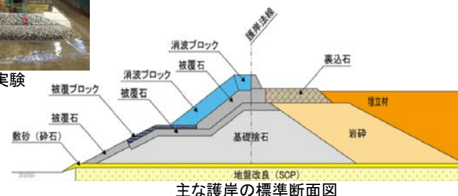
主要護岸の標準断面図
